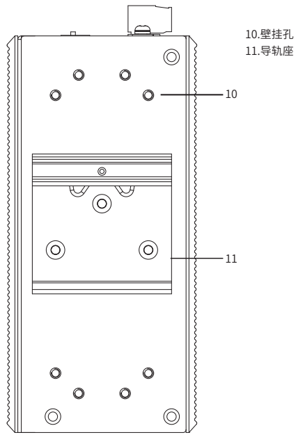
TL-SG2216工业级 后面板示意图
