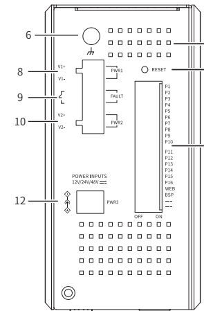
TL-SG2216工业级 上面板示意图
