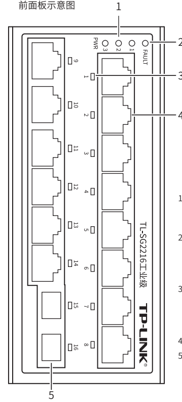
TL-SG2216工业级 前面板示意图
