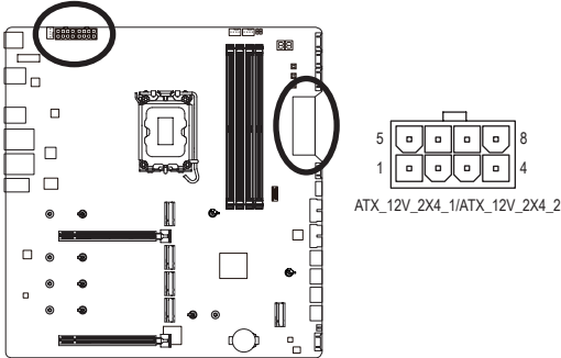
ATX_12V_2X4_1/ATX_12V_2X4_2 :
