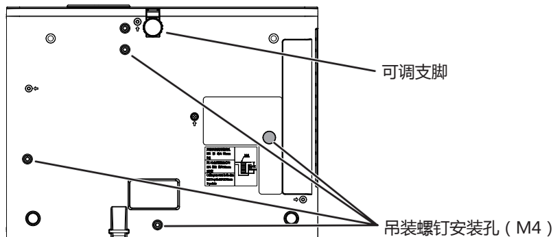
吊装螺钉安装孔和可调支脚的位置
